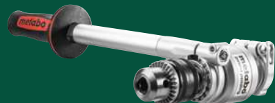
Triplicatore di coppia PowerX3 DC No.ord. 627232000
